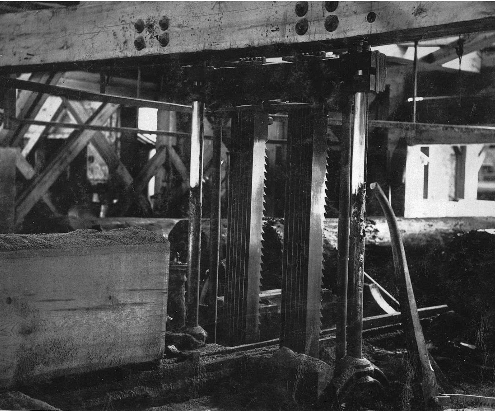
Figure 1.3 Une scie à châssis effectue simultanément plusieurs tranchages d'une bille de bois à la scierie Wright, Batson & Currier près d'Ottawa; musée McCord, 1872, William Notman, no d'accèsion 1-78896.1.
